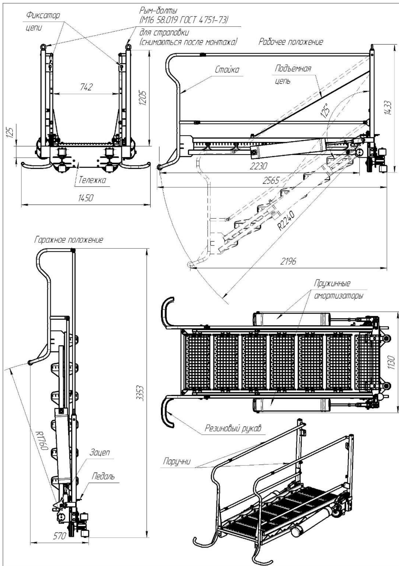
Габаритные размеры трапа 417.78.00.00.00-06 (-07) в рабочем и гаражном положениях
