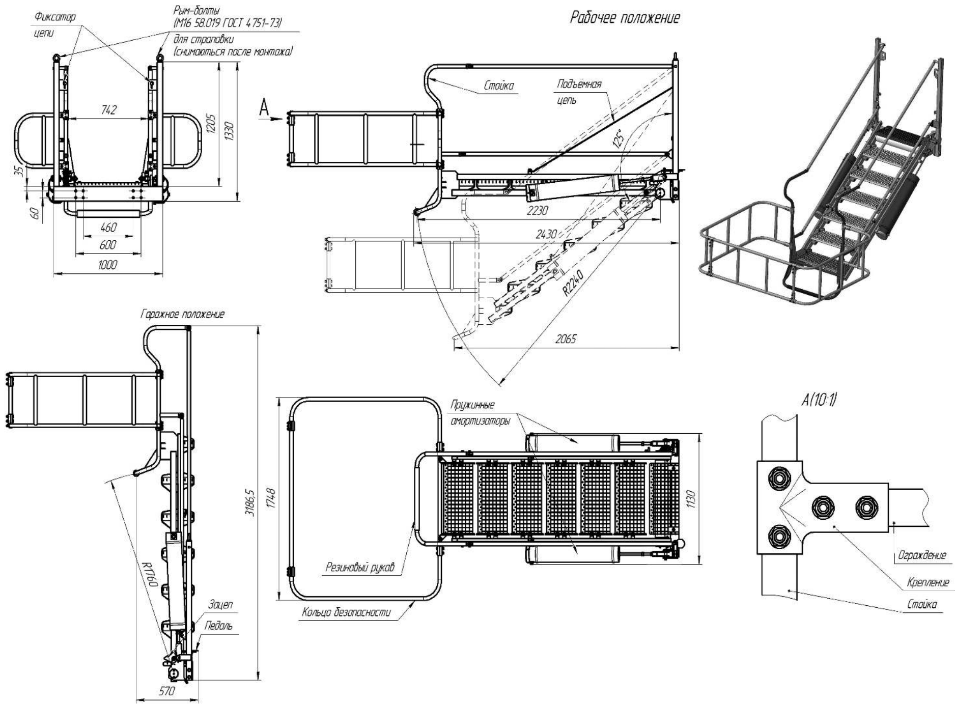
Габаритные размеры трапа 417.78.00.00.00-04(-05) в рабочем и гаражном положениях
