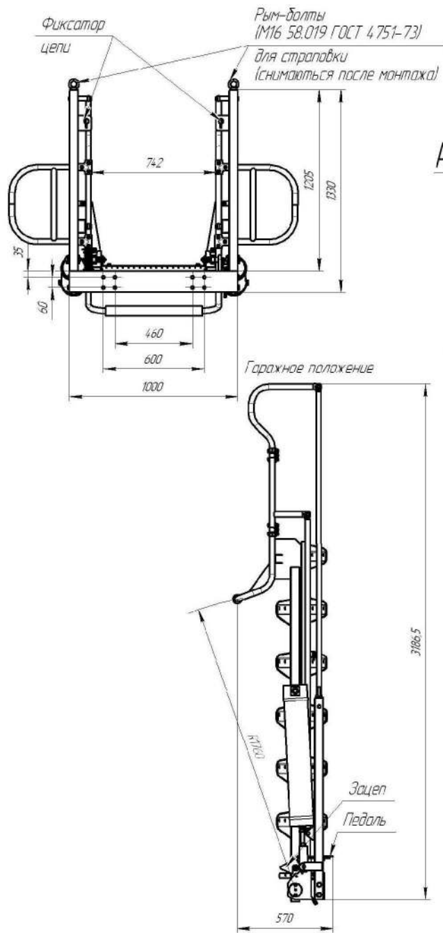
Габаритные размеры трапа 417.78.00.00.00-02 (-03) в рабочем и гаражном положениях
