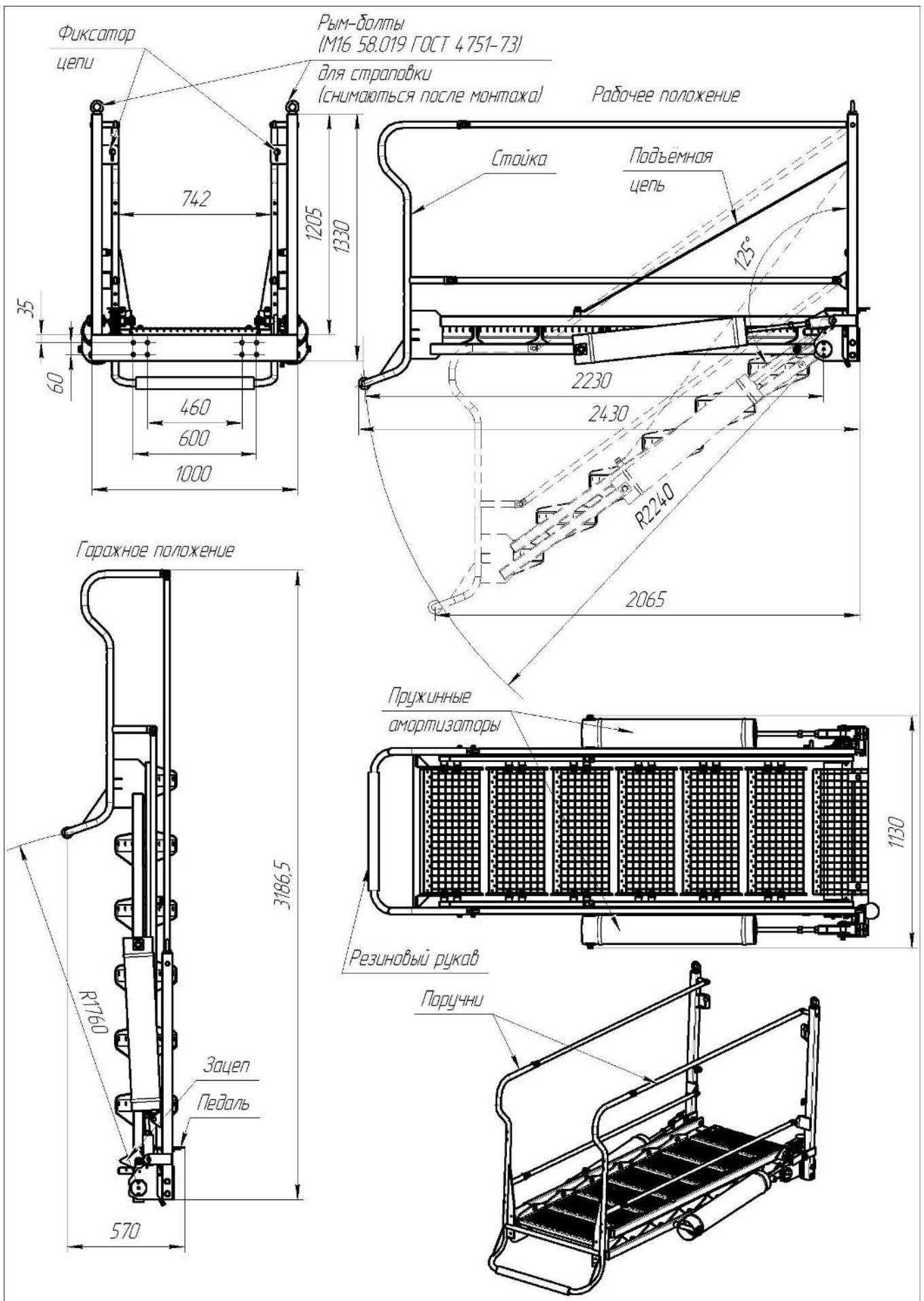
Габаритные размеры трапа 417.78.00.00.00 (-01) в рабочем и гаражном положениях
