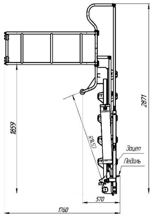
Габаритные размеры трапа 417.72.00.00.00-04 (-05) в рабочем и гаражном положениях
