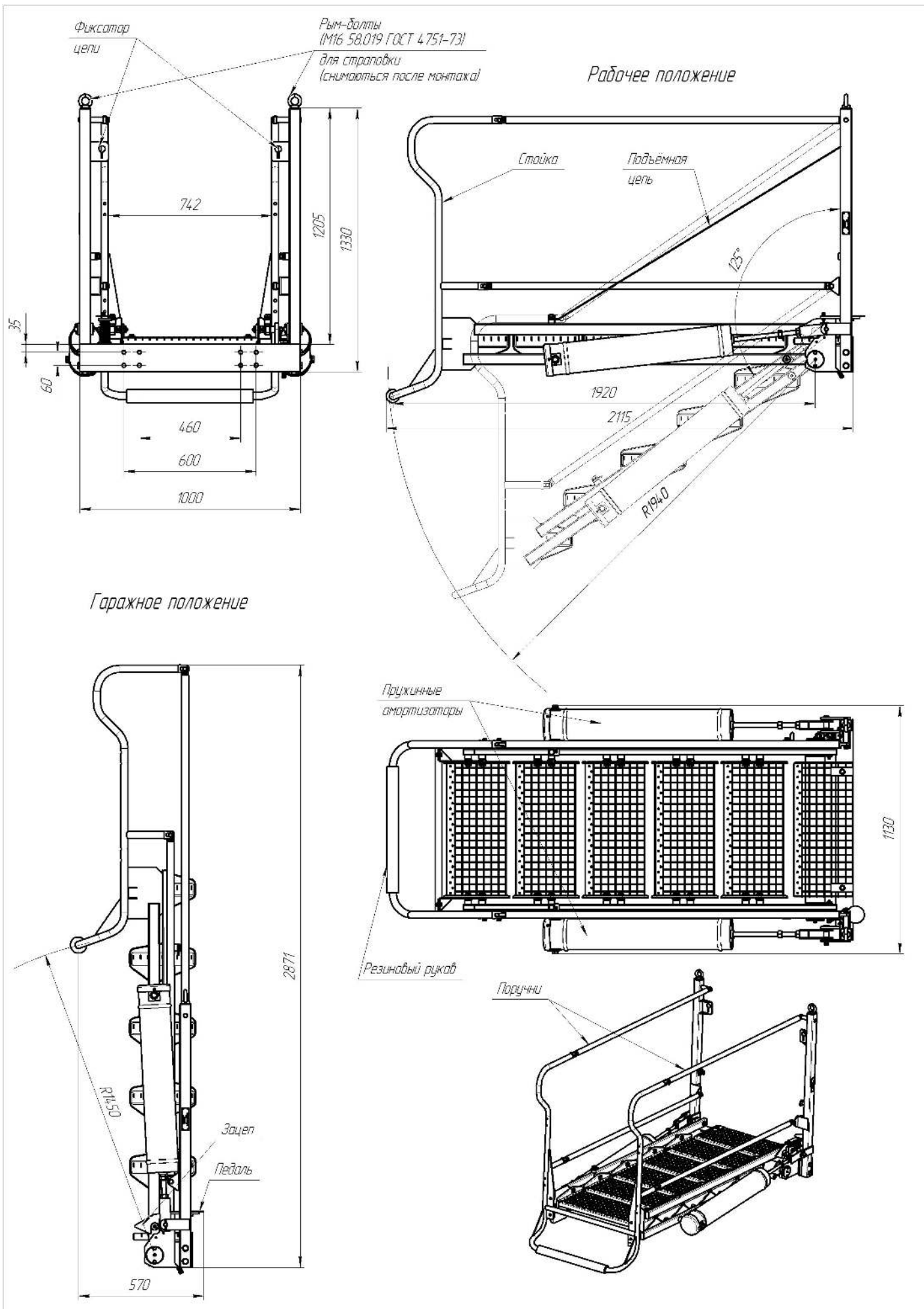
Габаритные размеры трапа 417.72.00.00.00 (-01) в рабочем и гаражном положениях
