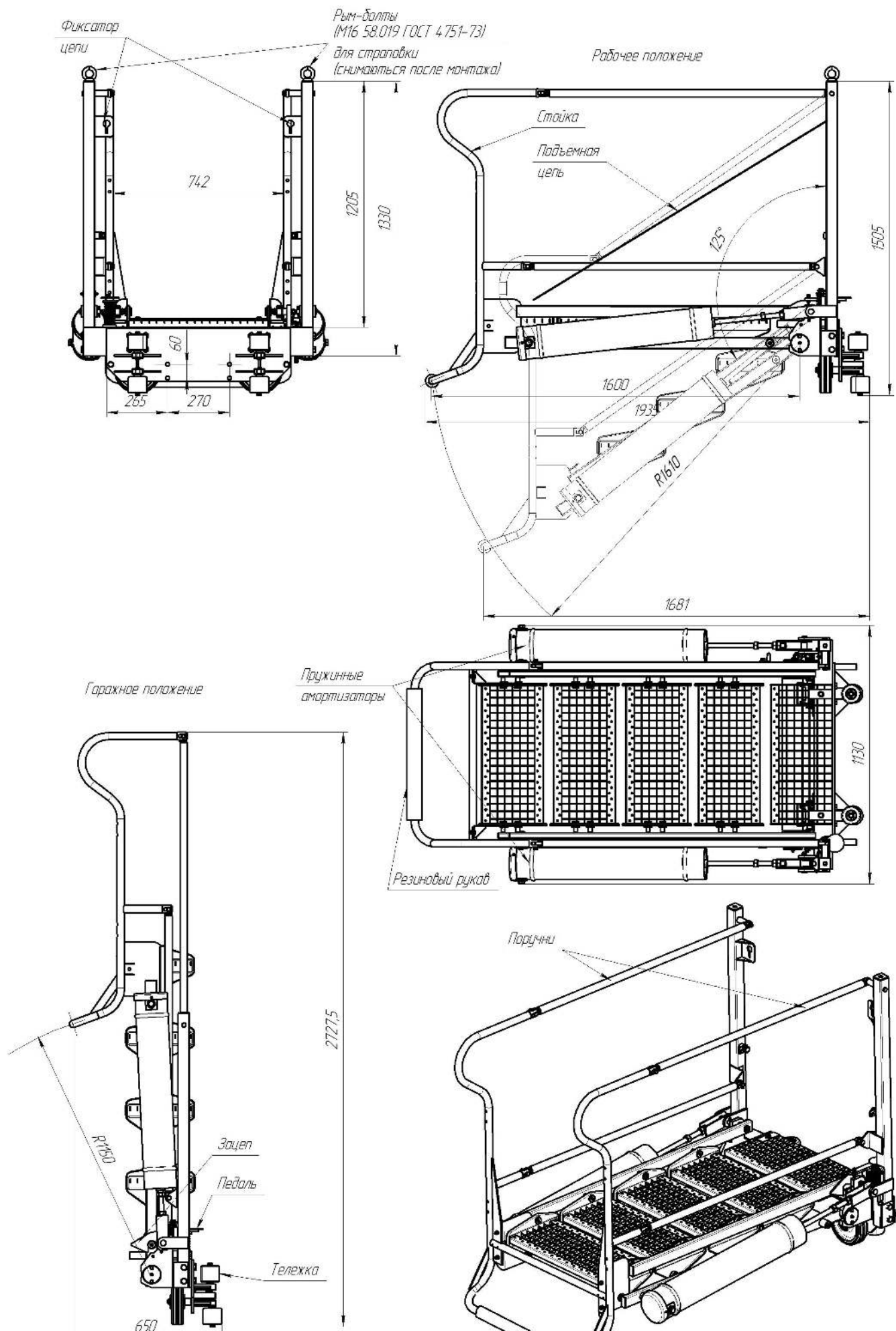
Габаритные размеры трапа 417.68.00.00.00-06 (-07) в рабочем и гаражном положениях
