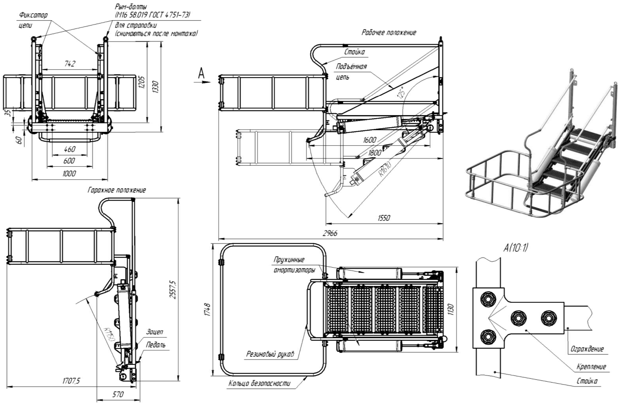
Рисунок А.3 - Габаритные размеры трапа 417.68.00.00.00-04 (-05) в рабочем и гаражном положениях
