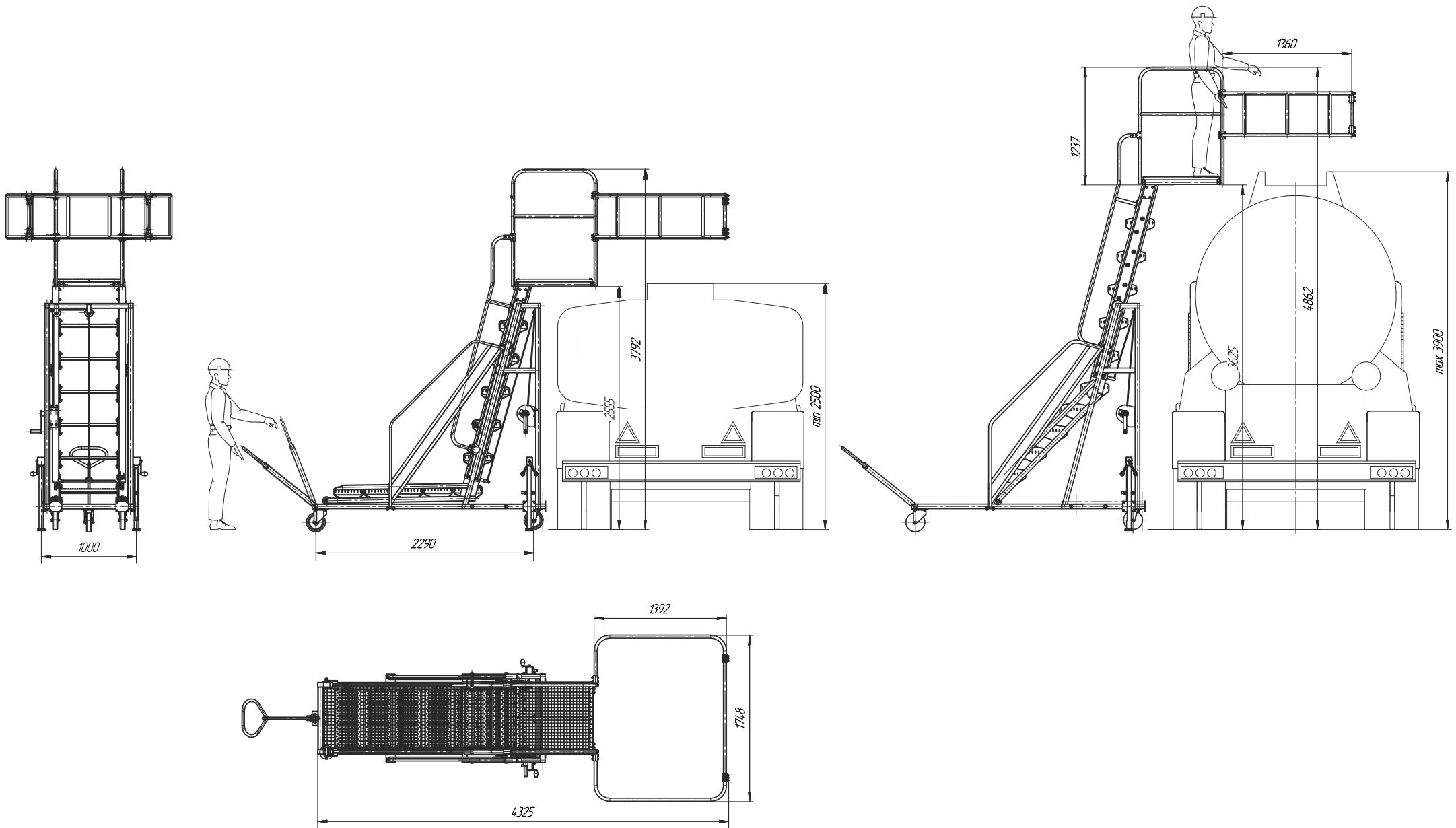
1220.00.00.00.00 Лестница передвижная для автоцистерн
